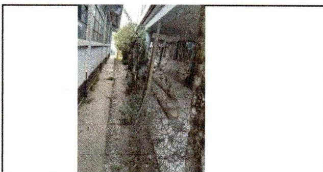
Foto 5: Reparacion de muro perimetral de block con tubo HG y malla galvanizada, soleras intermedias y columnas
